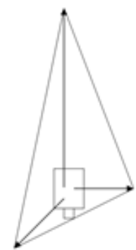
Ongelijkbenige driehoek
