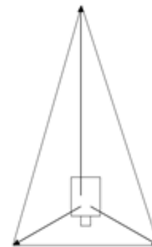
Gelijkbenige driehoek
